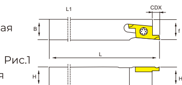
Державка-левая
