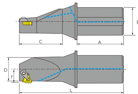
Державка-правая
