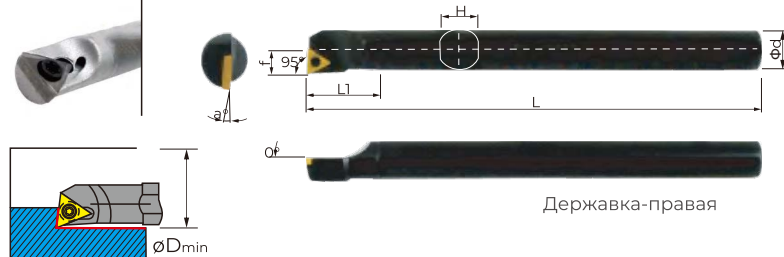
E..STUCR
