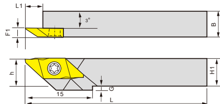
Державка-правая
