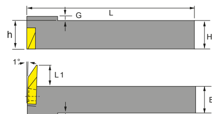
Державка-правая
