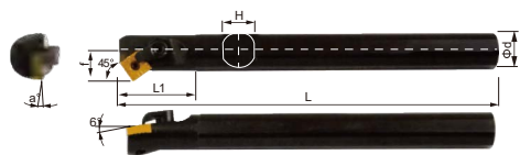
Державка-правая
