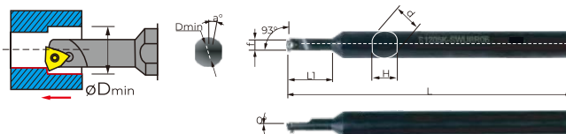
Державка-правая
