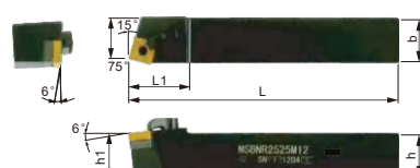
Державка-правая
