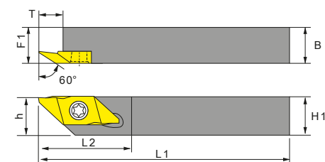
Державка-правая
