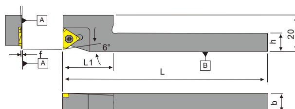
Державка-правая
