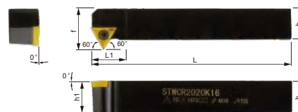
Державка-правая
