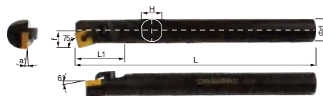
Державка-правая
