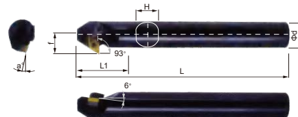
Державка-правая
