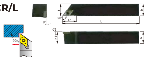
Державка-правая
