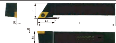
Державка-правая
