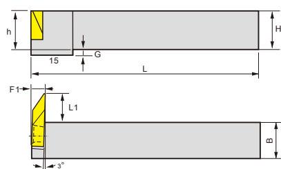
Державка-левая
