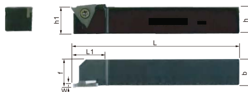
Державка-правая
