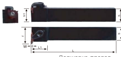
Державка-правая
