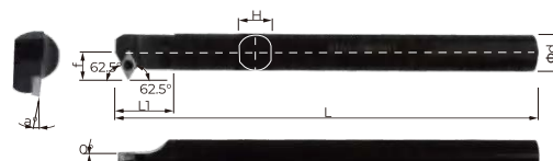
Державка-правая
