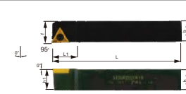
Державка-правая
