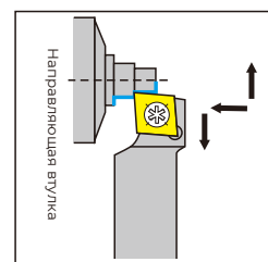
Державка-правая
