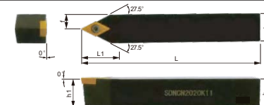
Державка-правая
