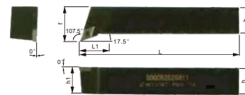
Державка-правая
