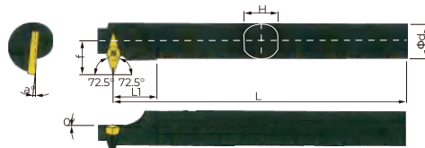
Державка-правая
