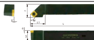
Державка-правая
