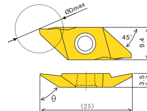
TBPA ØDmax=Ø5~12mm
