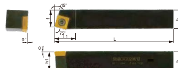
Державка-правая
